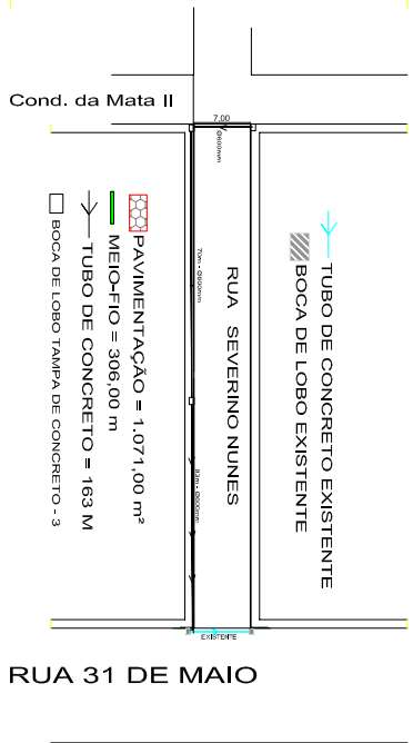
03 Projeto Pluvial Pavimentação Rua Severino Nunes
