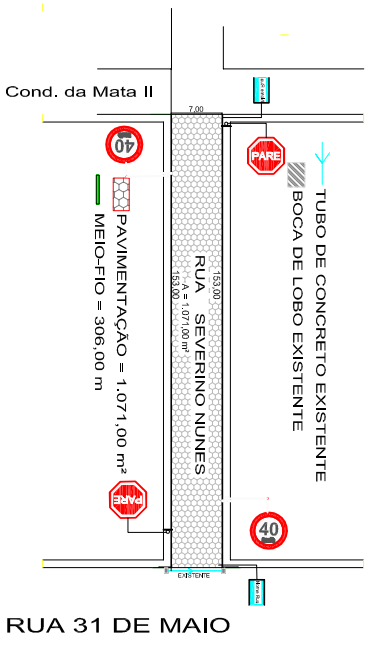
03 Projeto Sinalização Pavimentação Rua Severino Nunes
